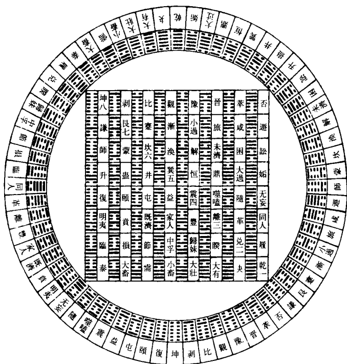
伏羲六十四卦方圆图
